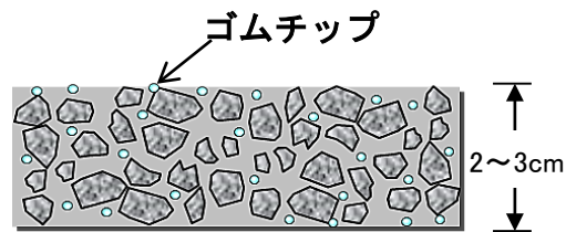
〔薄層シングルメルト概念図〕
