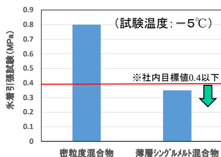
〔凍結抑制効果の例(氷着引張試験)〕
