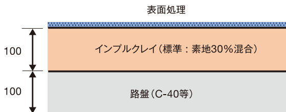
インブルクレイ工法の標準断面(例)
