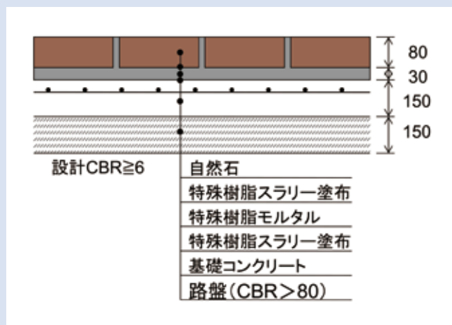
構内道路などの断面例
