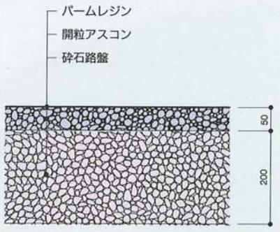
施工断面図
