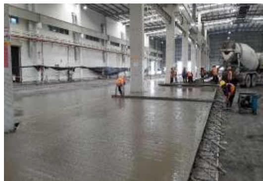
ブニアンチューブによるスラブコンクリート工事 人件費が安価なため人力施工が多いですが、品質は良好です。 【ドンナイ省】
