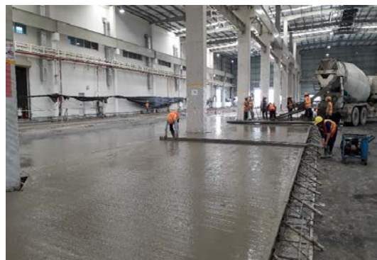
プニアンチューブによるスラブコンクリート工事 人件費が安価なため人力施工が多いですが、品質は良好です。 【ドンナイ省】
